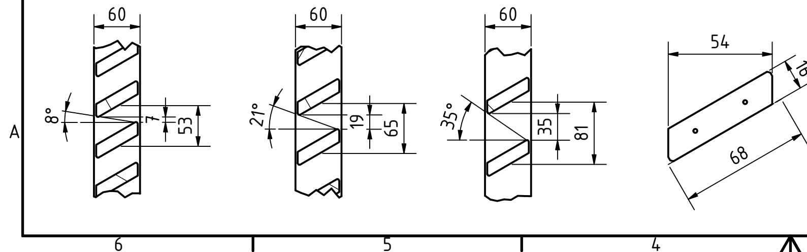
M ( 1 : 5 ) Standard center to center Fin Type
